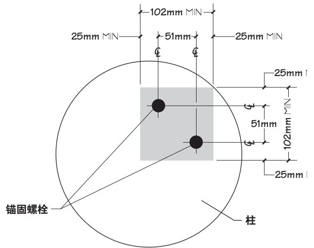
柱支撑细节
