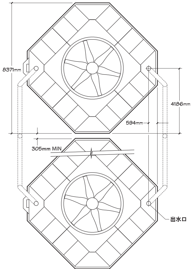
平面图 – 多间
