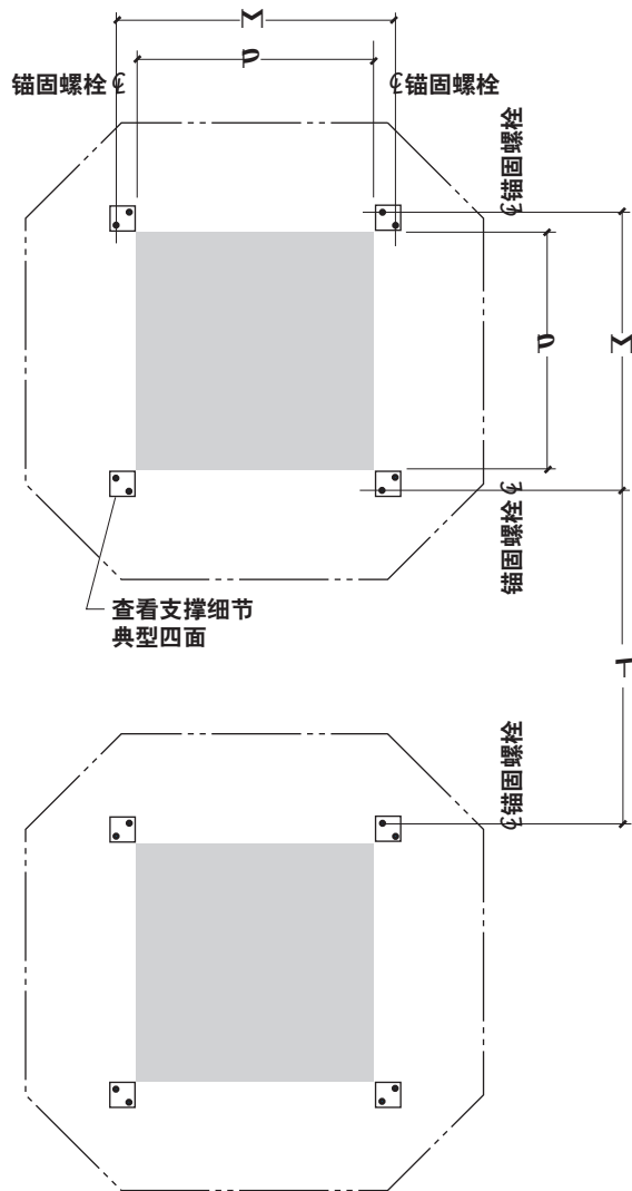
支撑平面图 – 两间
