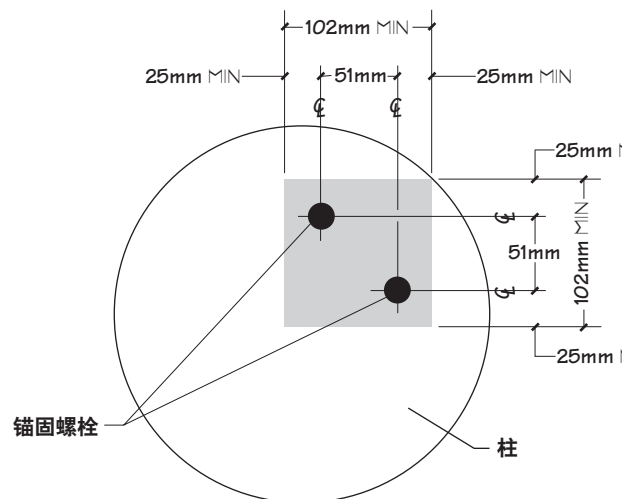
柱支撑细节
