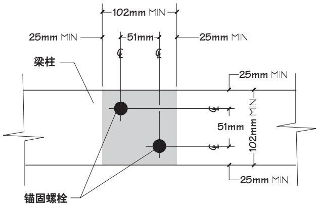
梁支撑细节
