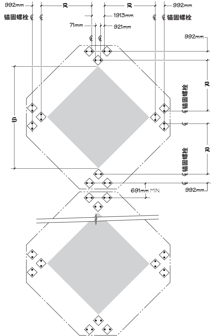
支撑平面图 - 多间
