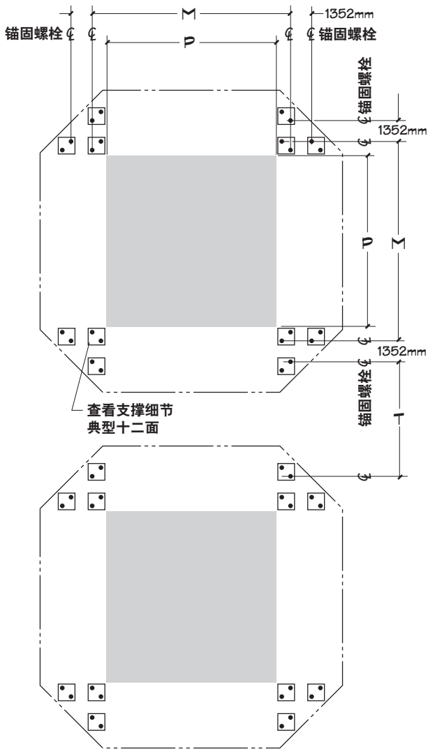
支撑平面图 - 两间
