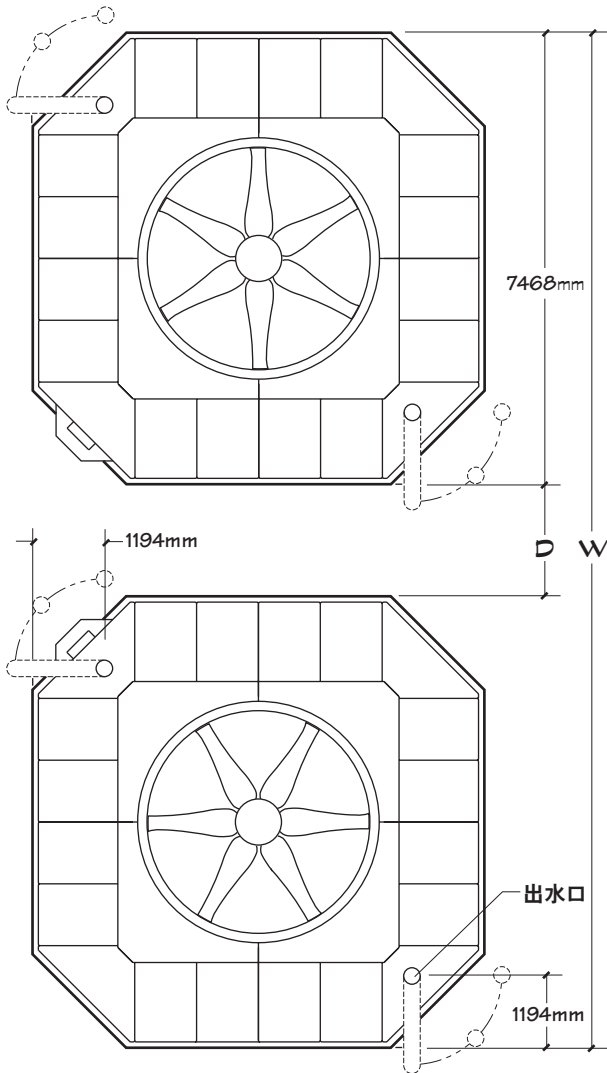
平面图 – 两间
