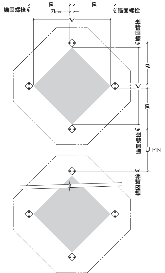
支撑平面图 – 多间
