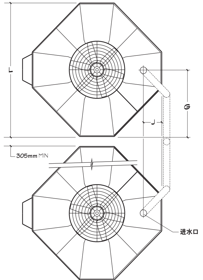
平面图 – 多间
