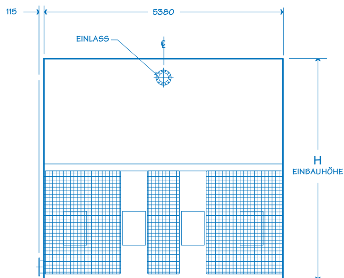
LUFTEINLASS-AUFRISS MODELLE 901956Q - 901959T
