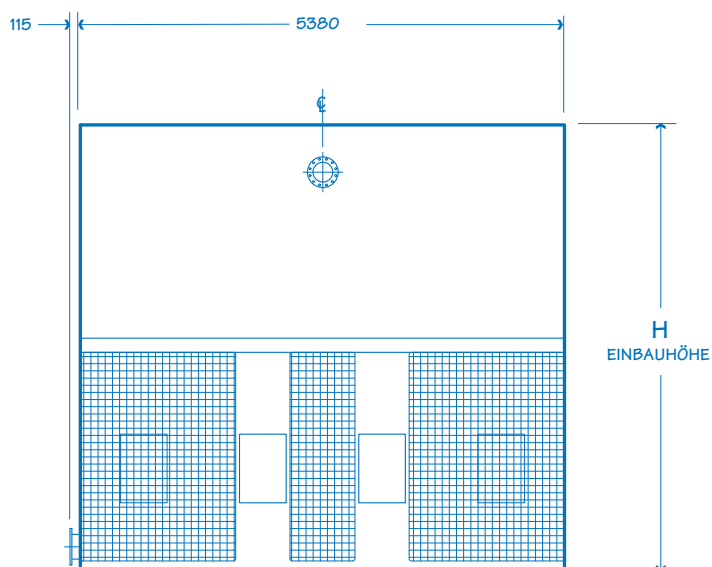
LUFTEINLASS-AUFRISS MODELLE 901556N - 901558R
