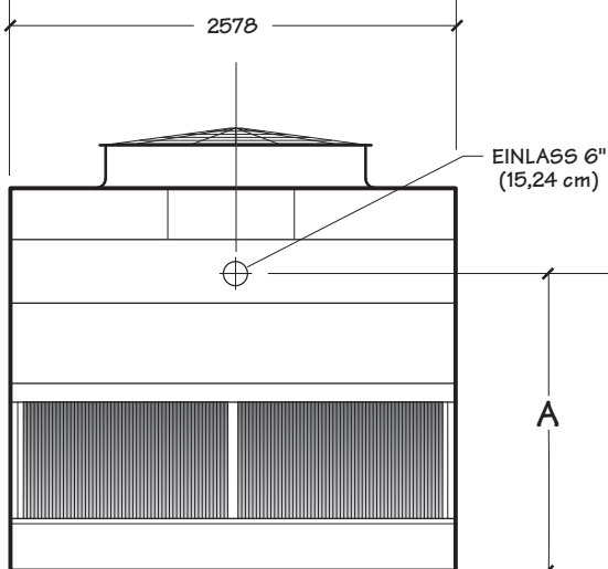
SEITENANSICHT LÄNGSSEITE
