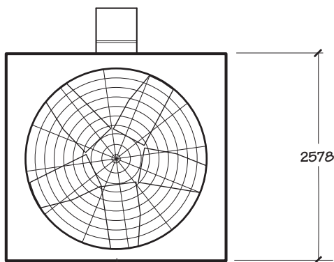
GRUNDRISS
