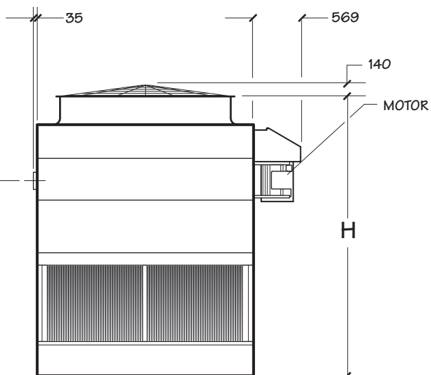
SEITENANSICHT BREITSEITE
