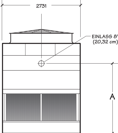
SEITENANSICHT LÄNGSSEITE
