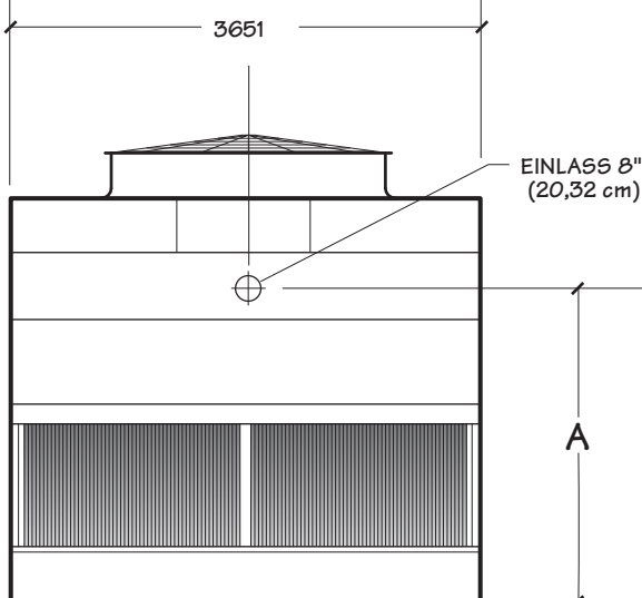
SEITENANSICHT LÄNGSSEITE
