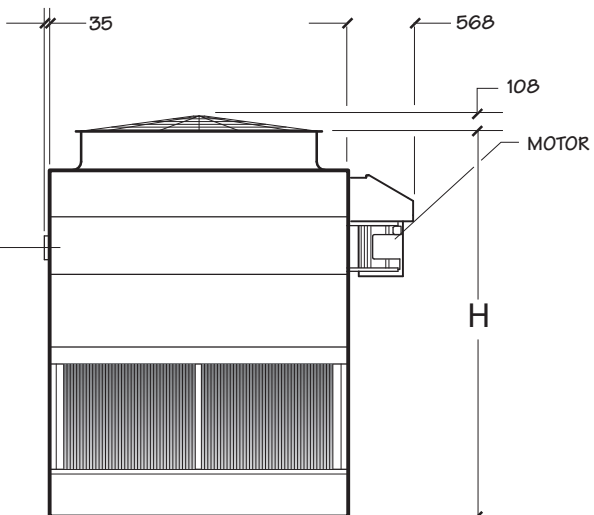
SEITENANSICHT BREITSEITE
