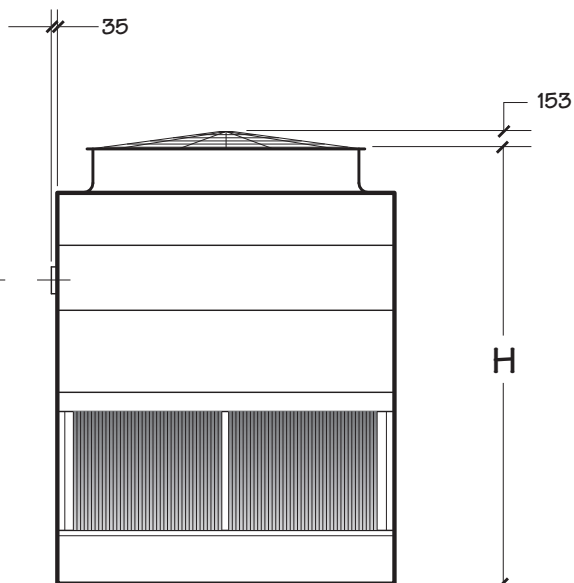
SEITENANSICHT BREITSEITE
