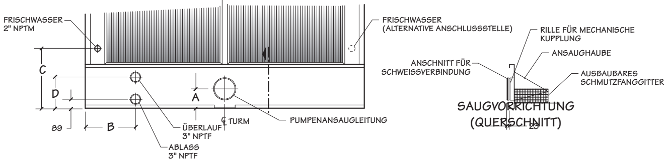
SAUGANSCHLUSS AN DER LÄNGSSEITE
