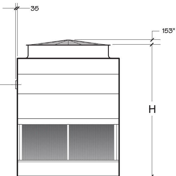
SEITENANSICHT BREITSEITE
