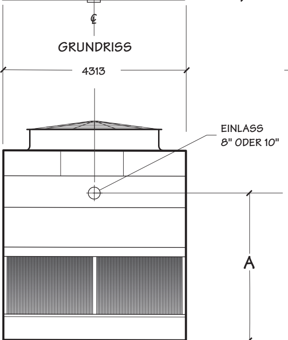
SEITENANSICHT LÄNGSSEITE
