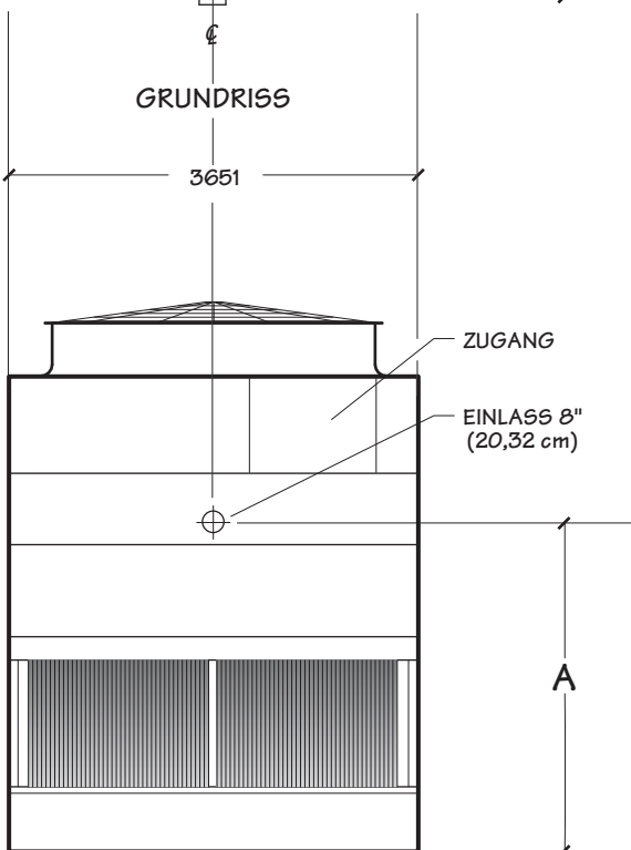
SEITENANSICHT LÄNGSSEITE
