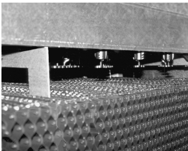
Капкоуловите със свалена гарнитура, за да се види зоната на разпределение чрез дюзи над пълнежа
