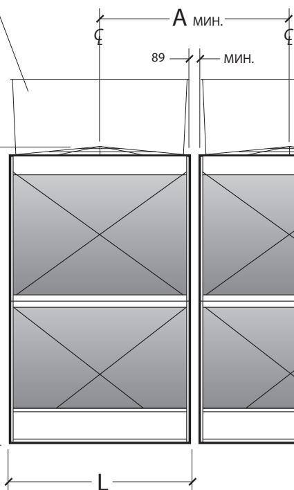
ИЗГЛЕД КЪМ ОТВОРА ЗА ПРИТОК НА ВЪЗДУХ
