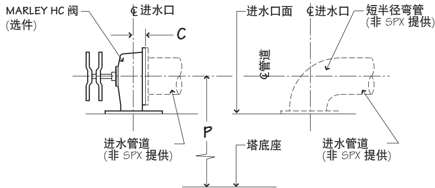
进水管道详细图
