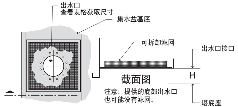
底部出水口接口
