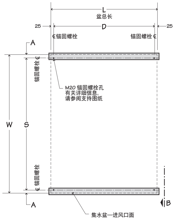
支撑钢架 选项二
