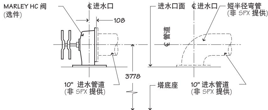
进水管详细详细信息
