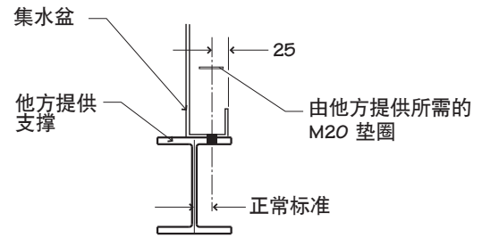
截面图 A
