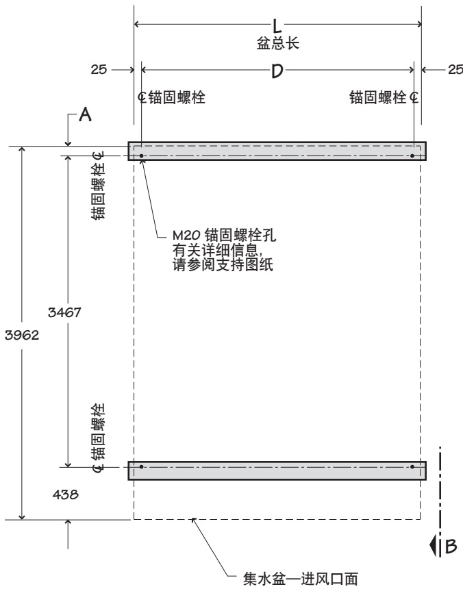
支撑钢架 选件三 6805 只要
