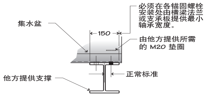
相对于横梁方向的锚固螺栓位置可选
