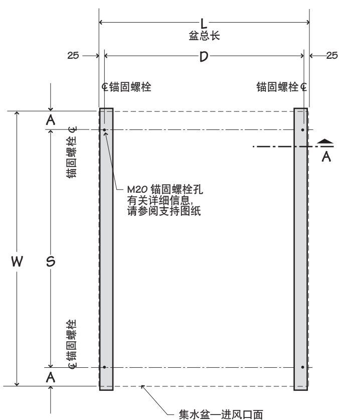
支撑钢架 选项一
