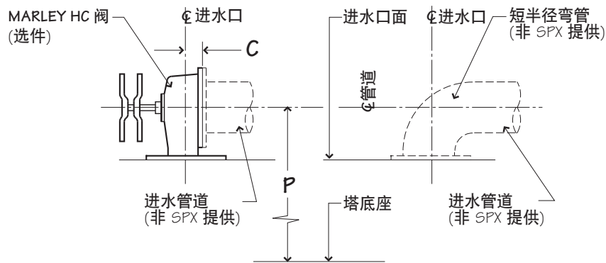
进水管详细信息
