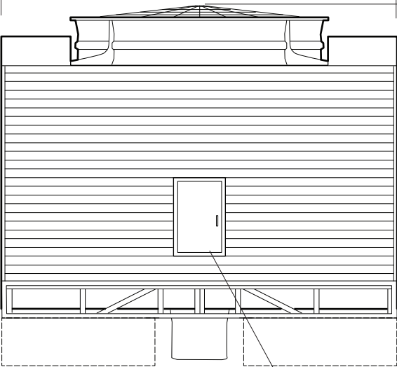
侧立面图
