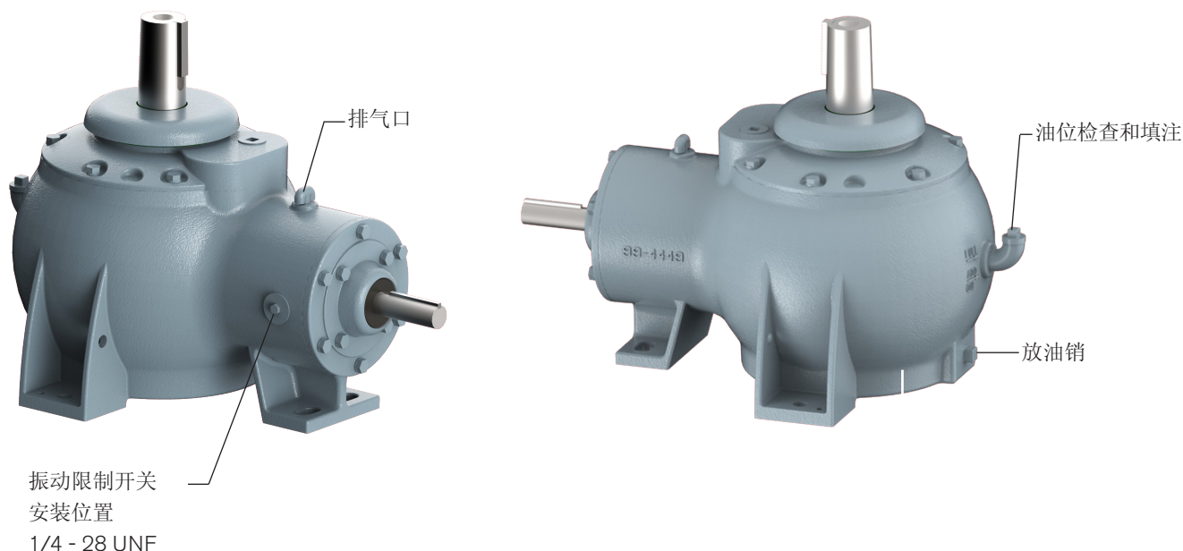
图 1 维修配件
