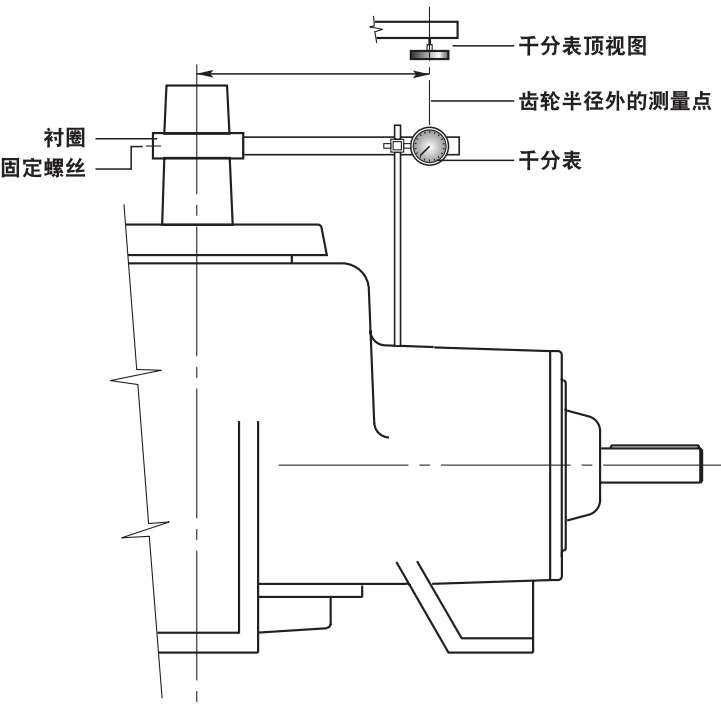
图 5 齿轮间隙测量
