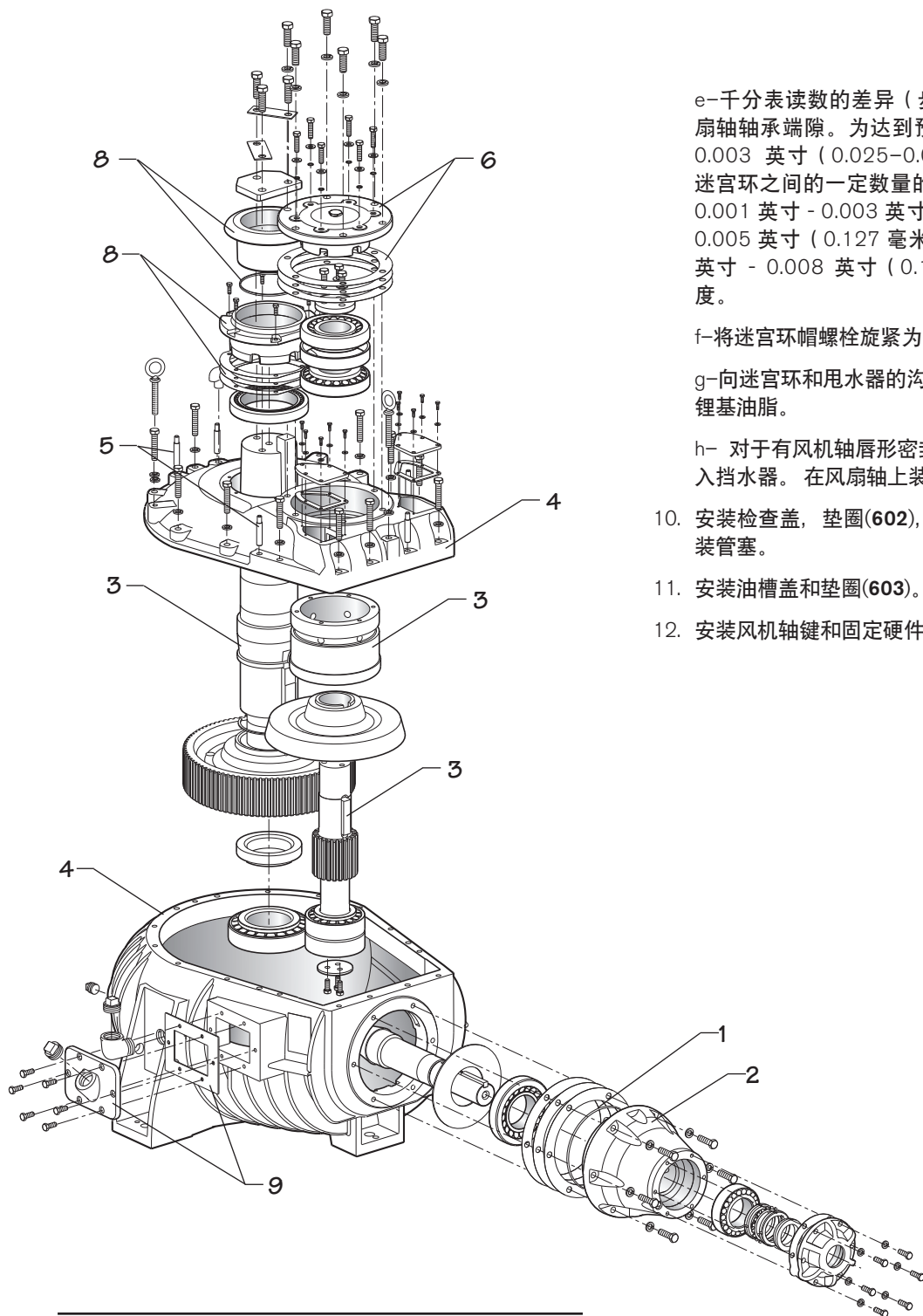
图 15 总装
