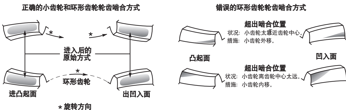
图 14 螺旋锥齿轮啮合方式
