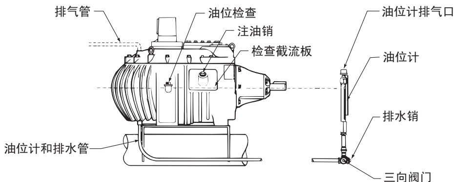
图 1 维修配件
