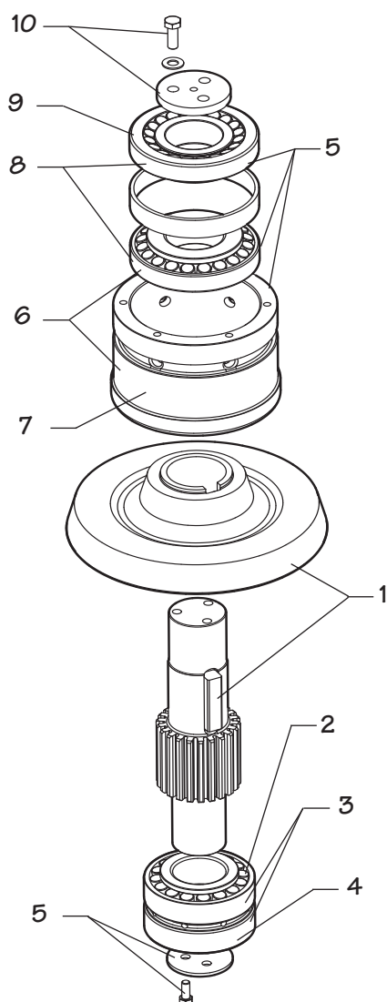
图 13 级间装配
