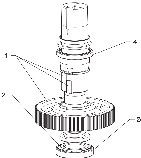
图 14 风扇轴装配
