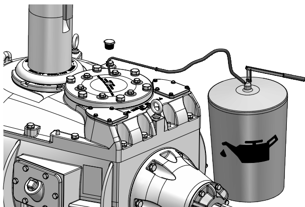
图 3 运行级间轴
