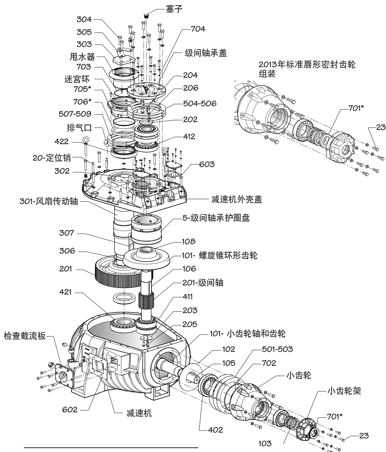
图 3 分解装配
