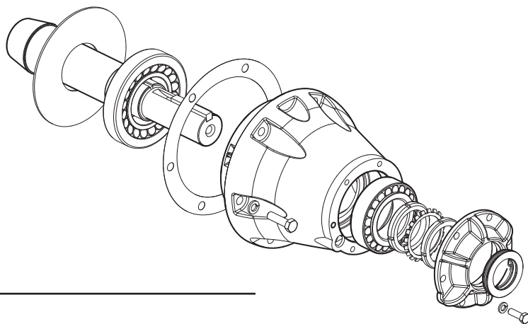
图 8 小齿轮架的拆卸
