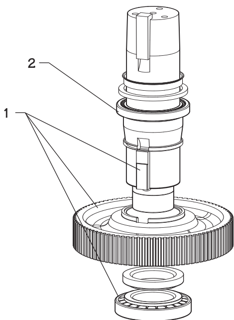
图 10 风扇轴的拆卸
