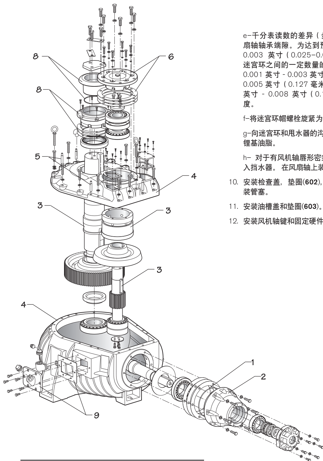
图 15 总装
