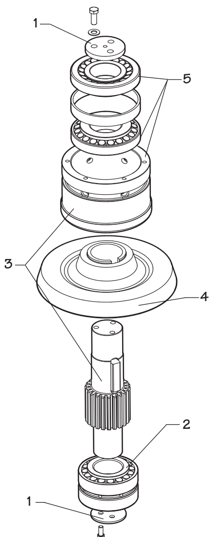
图 9 级间的拆卸
