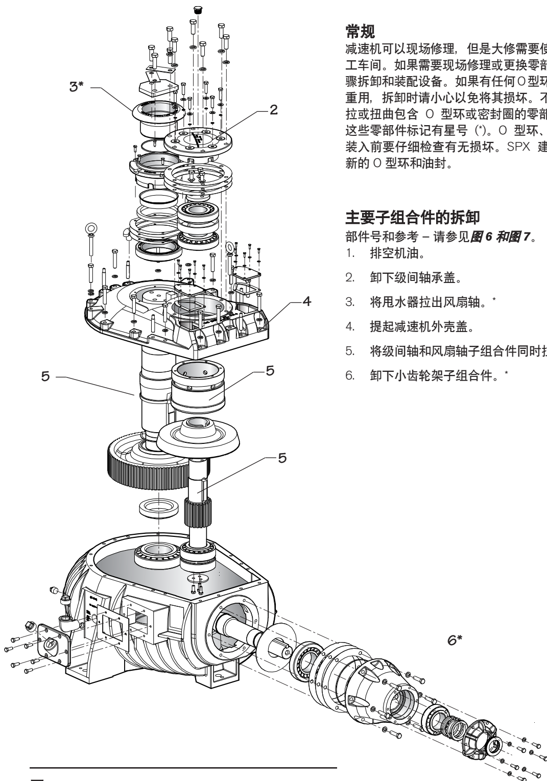
图 7 主要子组合件的拆卸
