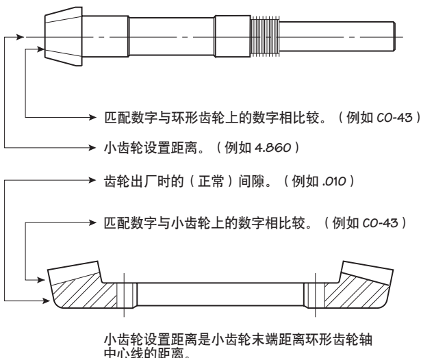
图 11 齿轮匹配数字和设置数据
