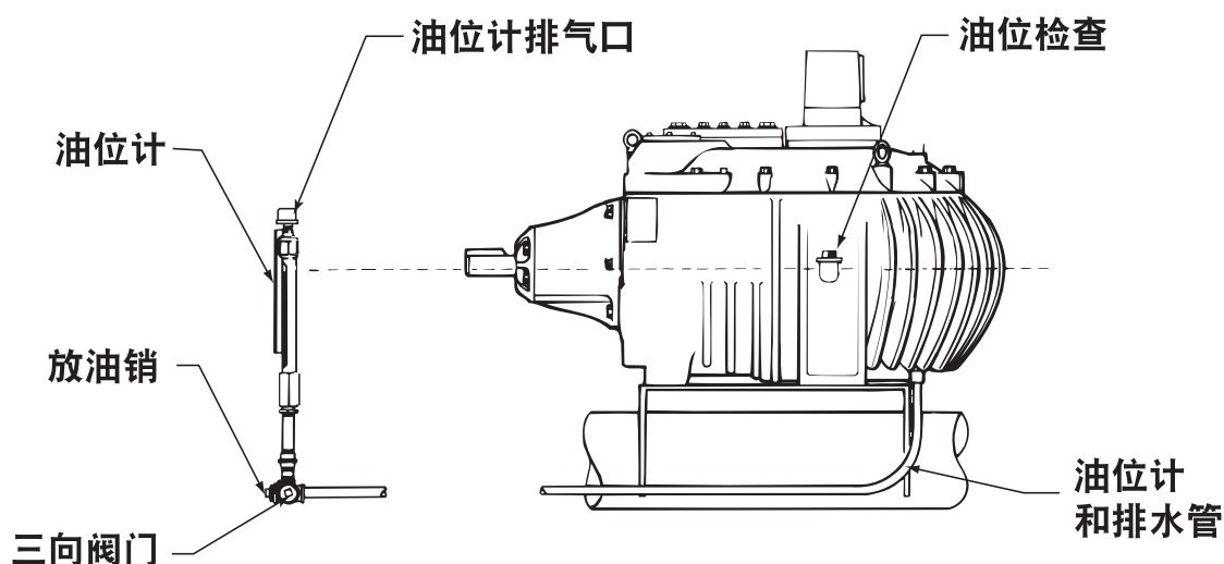
图 2 - 维修配件
