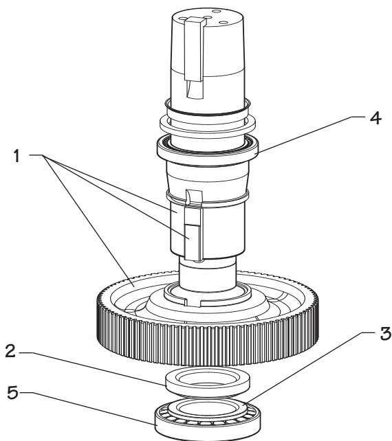
Bild 12 Lüfterwellen-Baugruppe
