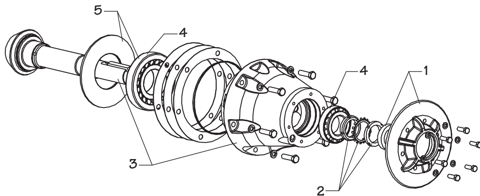
Bild 6 Demontage des Pleuellwellenkäfigs
