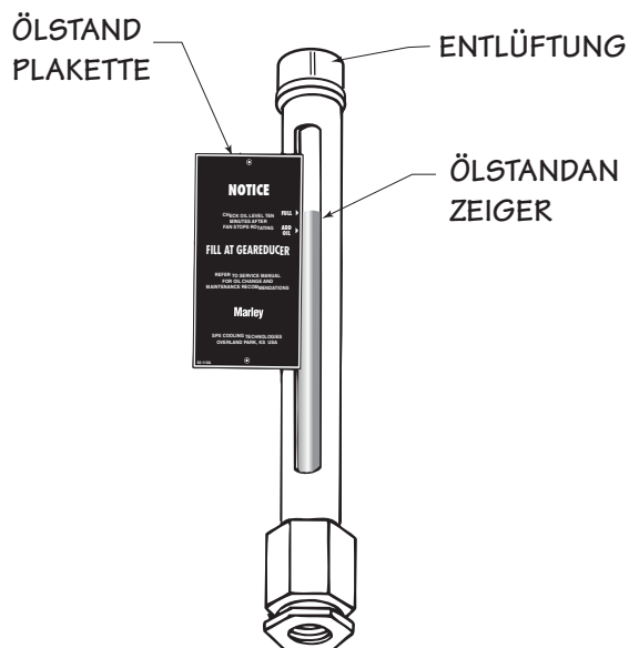
Abbildung 3 Montage des Ölstandanzeigers
