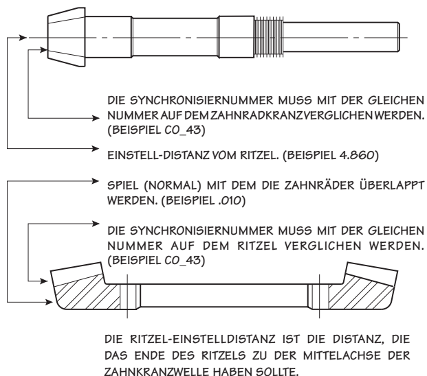
Bild 9 Zahnrad-Synchronisierungsnummern und Einstell-Daten
