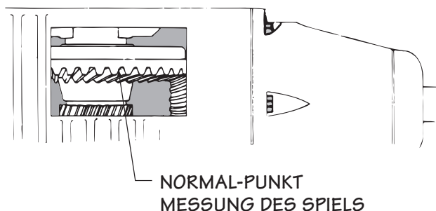
Bild 14 Messung des Radlager-Spiels
