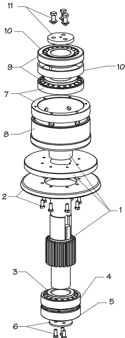
Bild 11 Zwischenstufe-Baugruppe
