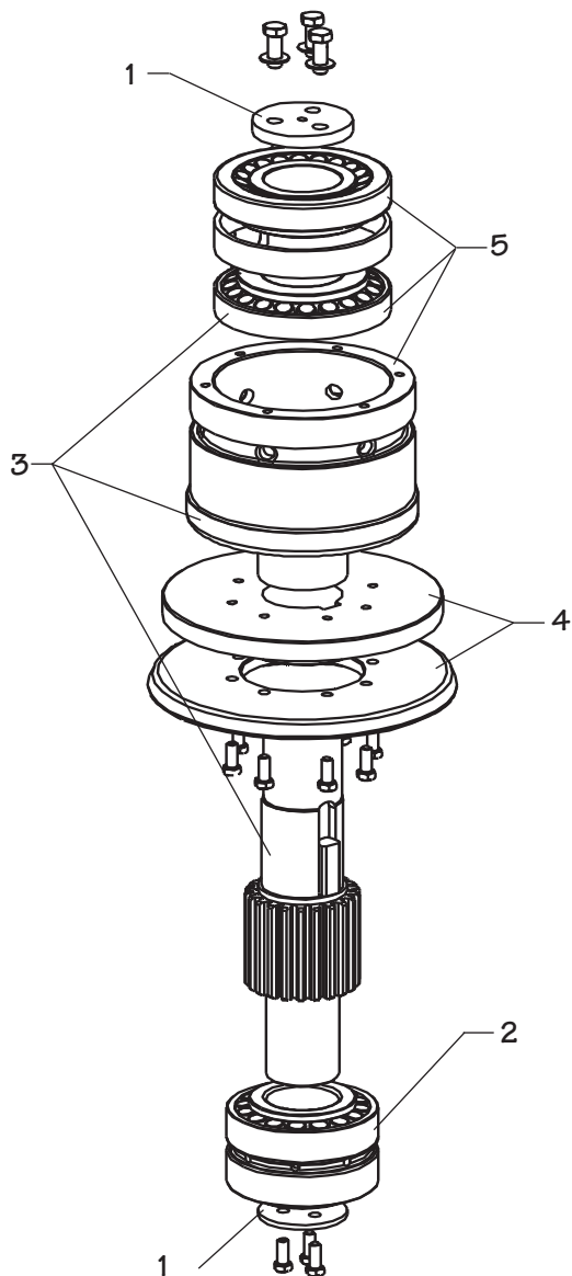
Bild 7 Demontage der Zwischenstufe
