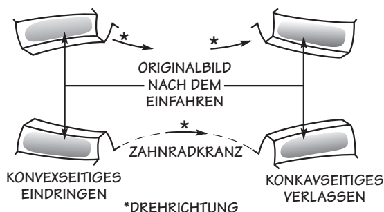
Bild 15 Verzahnungsbild des Spiralkegelzahnrad
