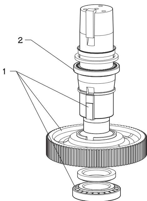
Bild 8 Demontage der Lüfterwelle
