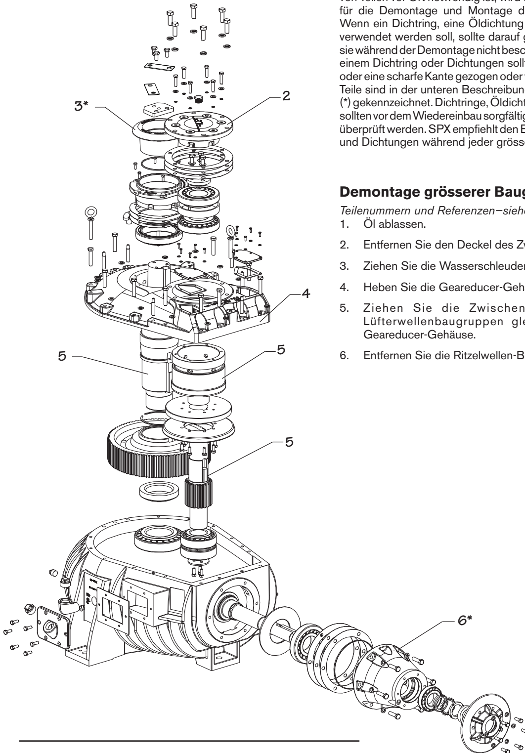
Bild 5 Demontage grösserer Baugruppen
