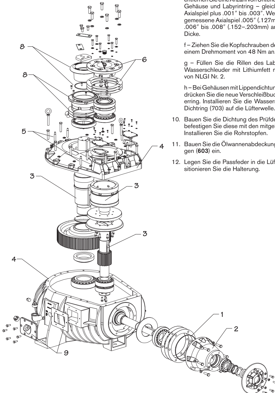
Bild 13 Endmontage
