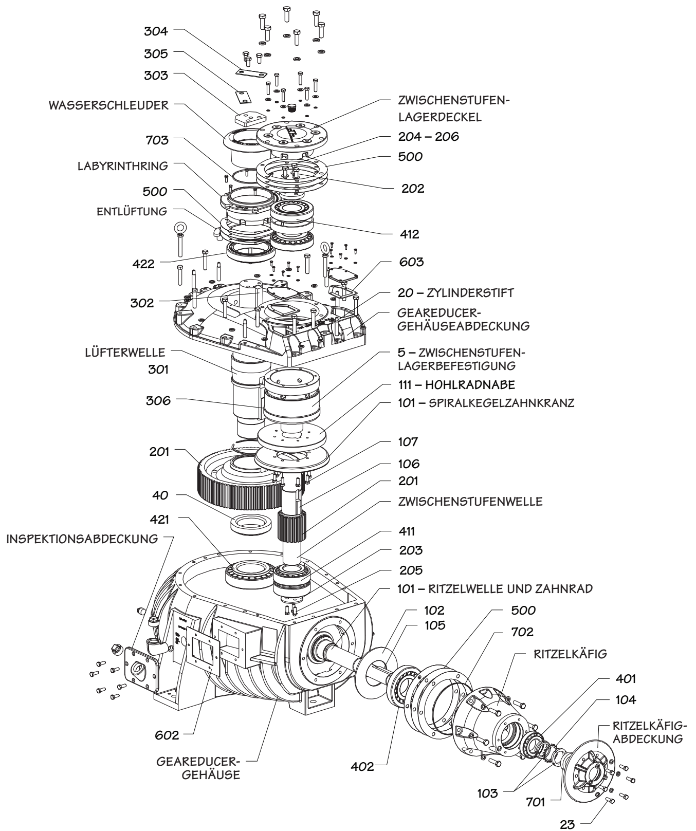
Bild 4 Explosionszeichnung
