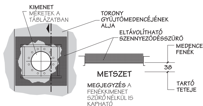
FENÉKKIMENET CSATLAKOZÁSA
