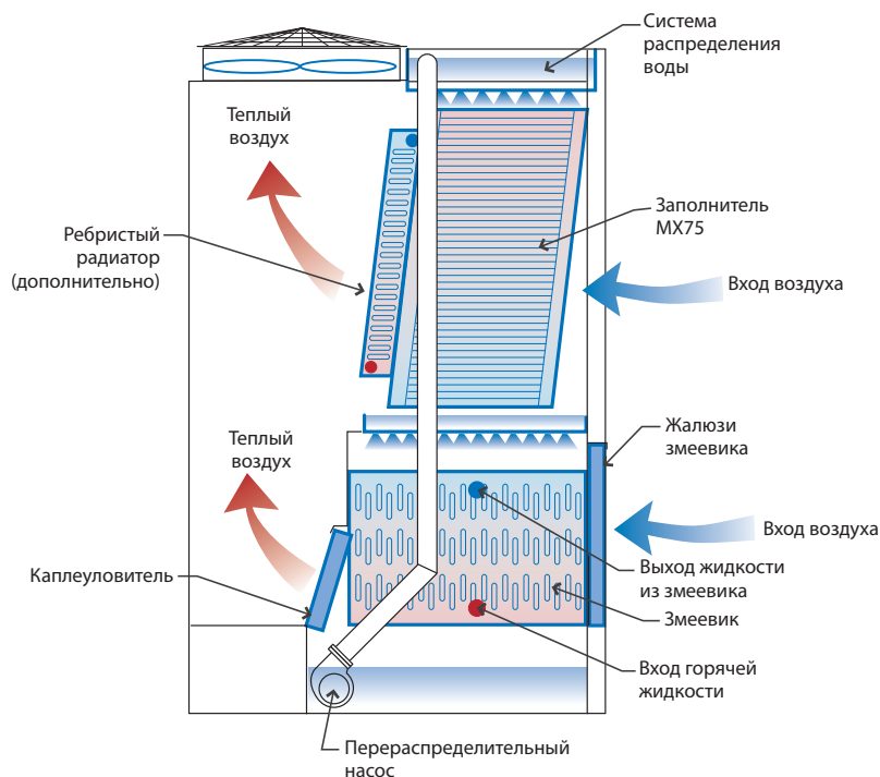
Опция Сухой охлаждения на моделях MNF7103, MNF7105 и MNF7107
