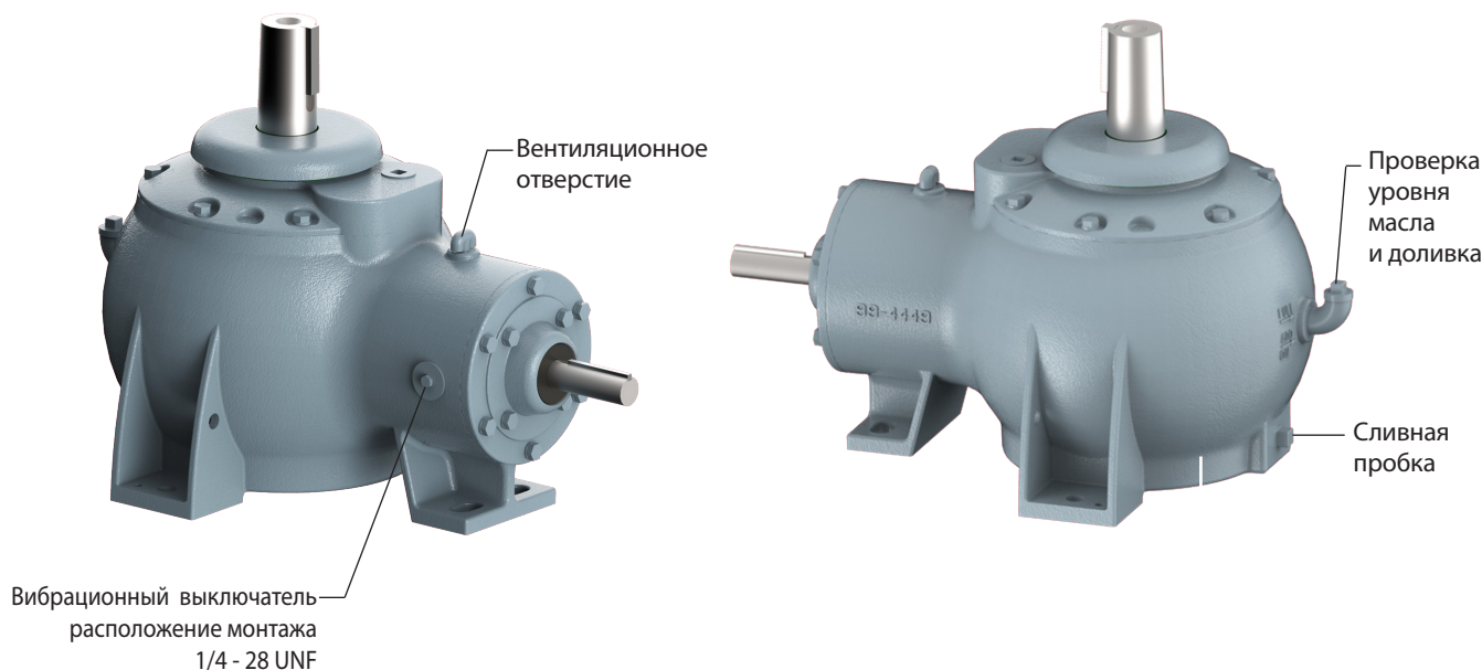
Рис. 1. Служебные фитинги
