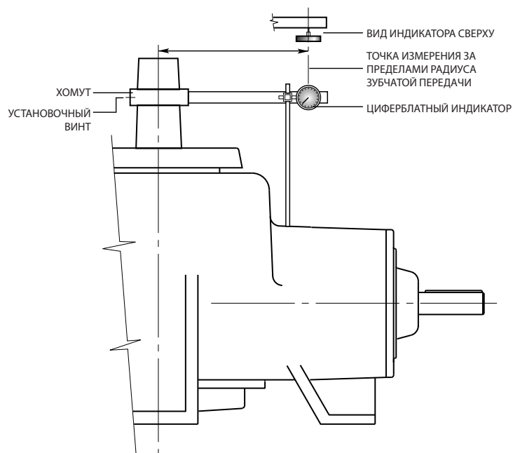
Рис. 5. Измерение зазора шестерен
