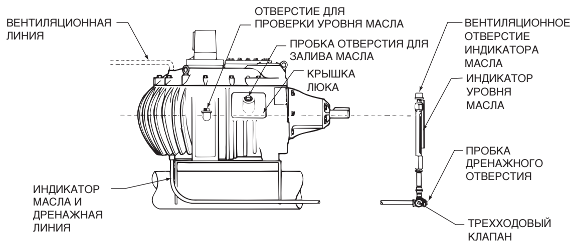
Рисунок 4 Службные фитинги
