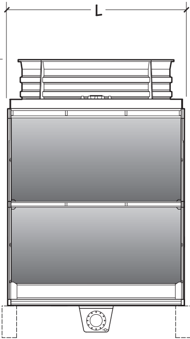
ELEVACIÓN DE ENTRADA DE AIRE
