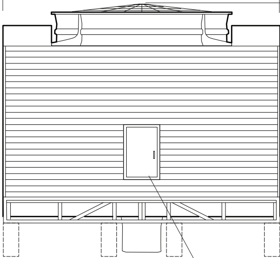
ELEVACIÓN LATERAL
