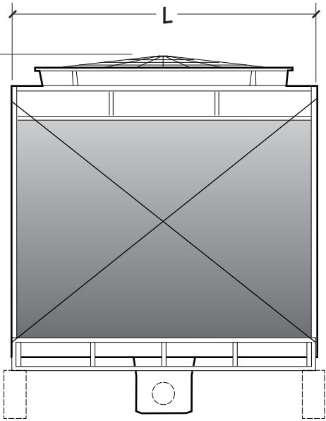
ELEVACIÓN DE ENTRADA DE AIRE
