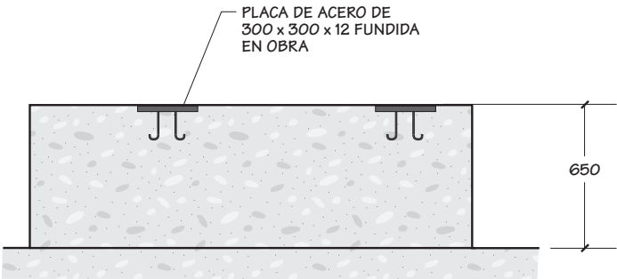
SECCIÓN B
