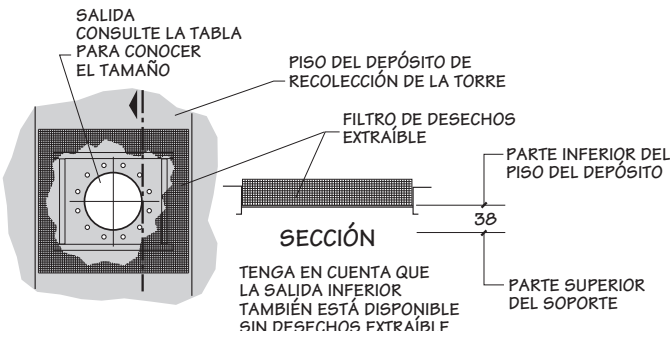
CONEXIÓN DE SALIDA INFERIOR
