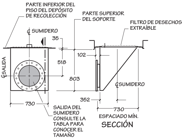
BRIDA CONEXIÓN DEL SUMIDERO DE SALIDA LATERAL CON DEPRESIÓN 16" Y 18" DIÁMETRO
