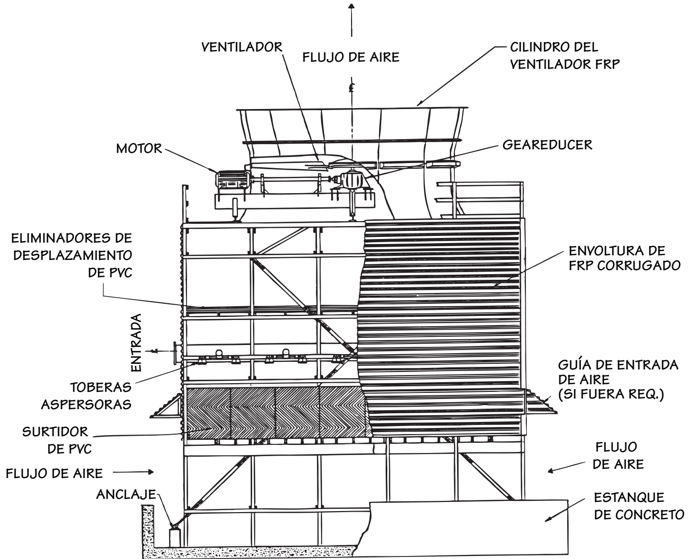
SECCIÓN TRANSVERSAL
